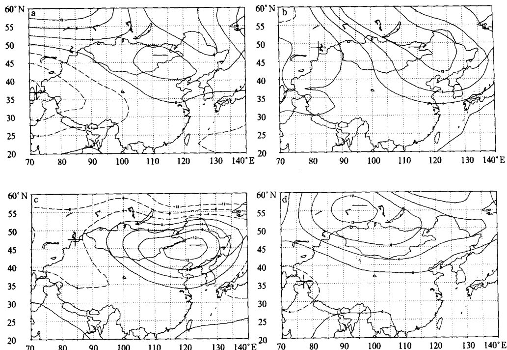
图 2 2002 年 3 月第 4 候(a),5 候(b)和 4 月第 2 候(c),3 候(d)500 hPa 高度距平场 (图中实线为负距平,虚线为正距平)
